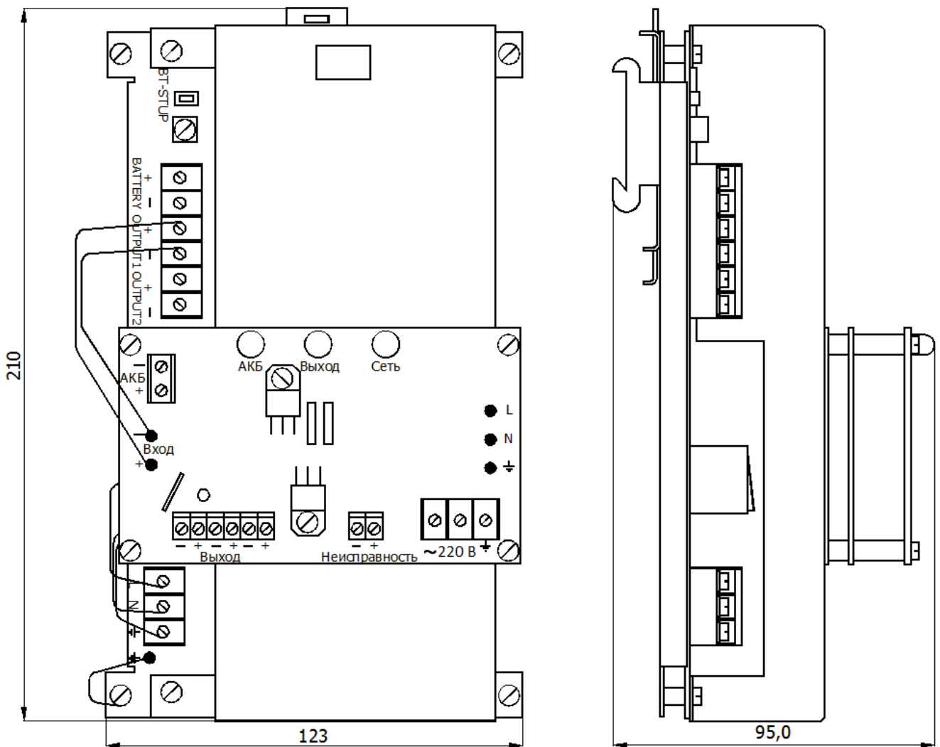
Рисунок 1 - Общий вид БРП
